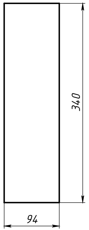
Поз.2 (Стойка)
