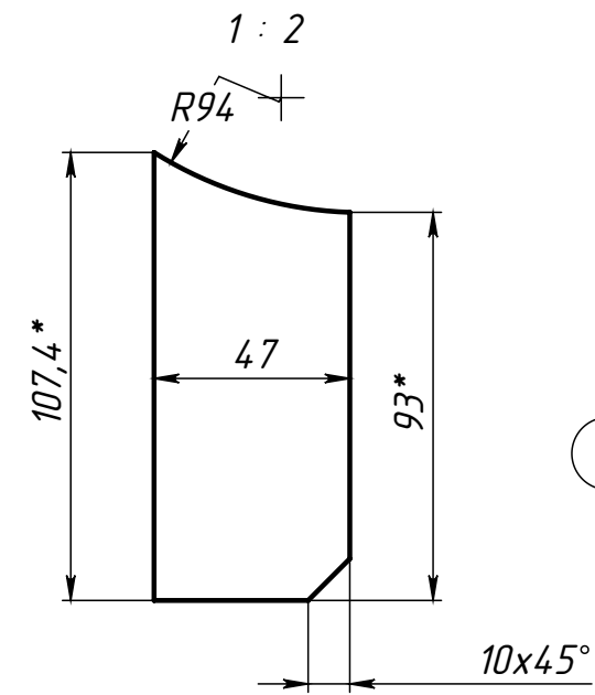
Поз.4 (Ребро)
