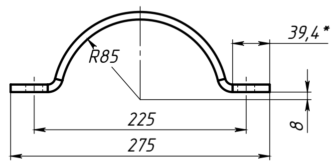
Поз.3 (Полухомут)
